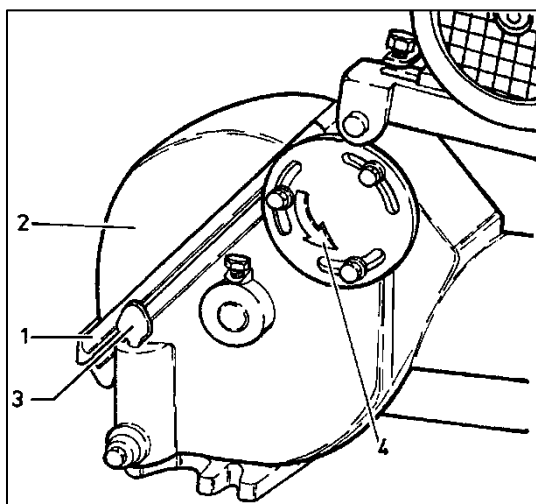
Abbildung 17: Antriebsgehäuse der Kolbenpumpe LG
