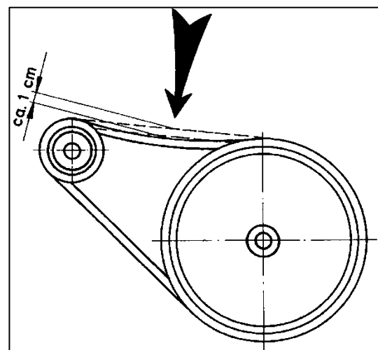
Abbildung 13: Keilriemen spannen
