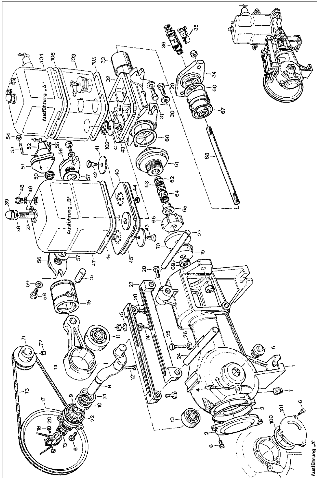
Abbildung 29: Explosionszeichnung der Kolbenpumpe L
