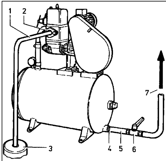
Abbildung 11: Wasseranschluss
