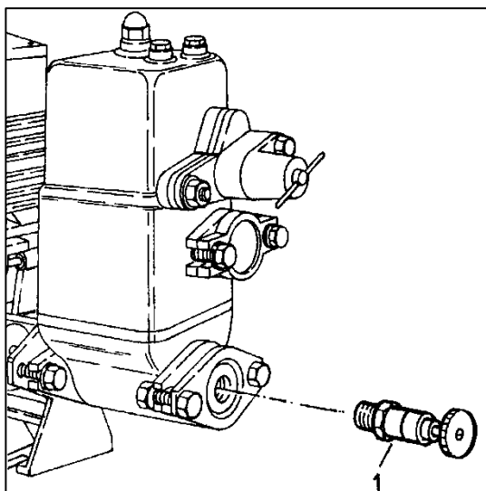
Abbildung 15: Schnüffelventil
