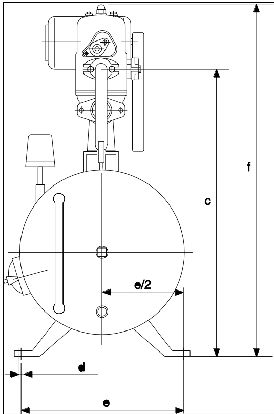
Abbildung 5: Maße in der Vorderansicht
