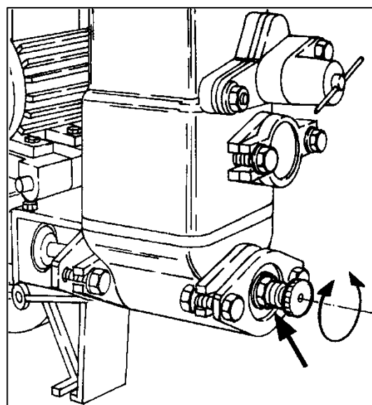
Abbildung 25: Luftpolsterergänzung
