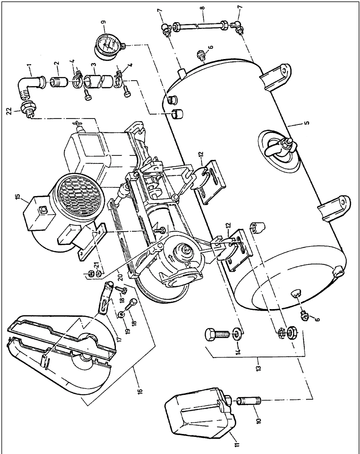
Abbildung 31: Explosionszeichnung des Hauswasserautomaten
