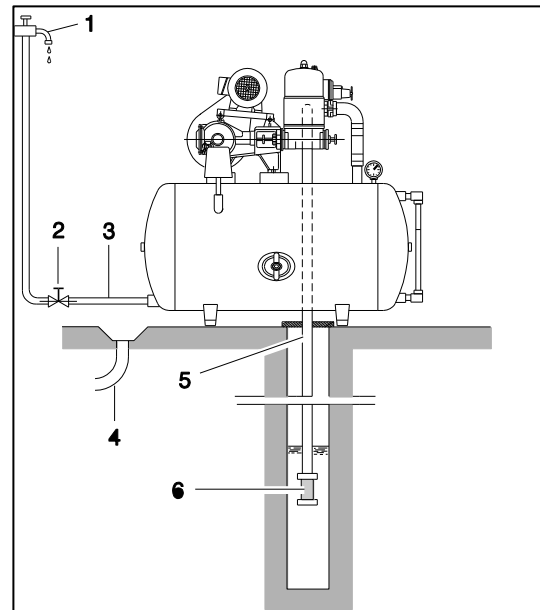
Abbildung 7: Aufbau des Hauswasserautomaten
