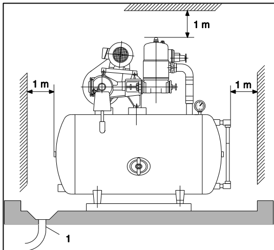
Abbildung 8: Aufstellraum Seitenansicht
