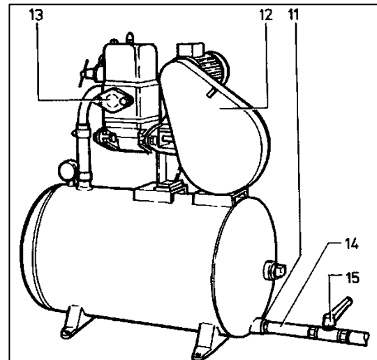
Abbildung 4: Funktionselemente 2
