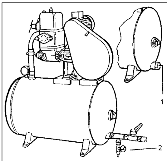
Abbildung 22: Automat entleeren
