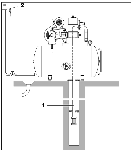
Abbildung 20: Anfahren des Hauswasserautomaten
