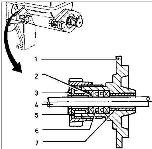
Abbildung 26: Stopfbuchse
