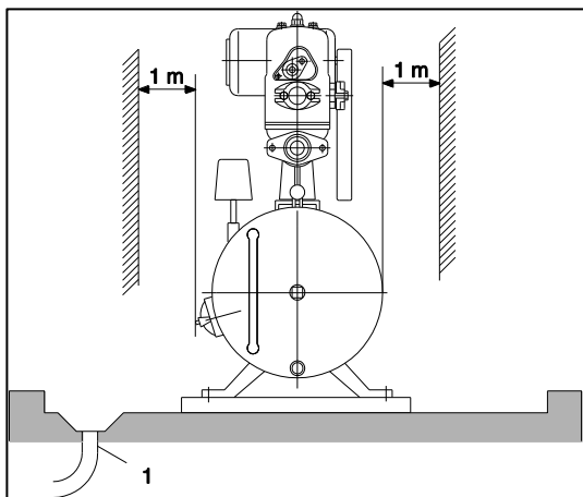
Abbildung 9: Aufstellraum Vorderansicht
