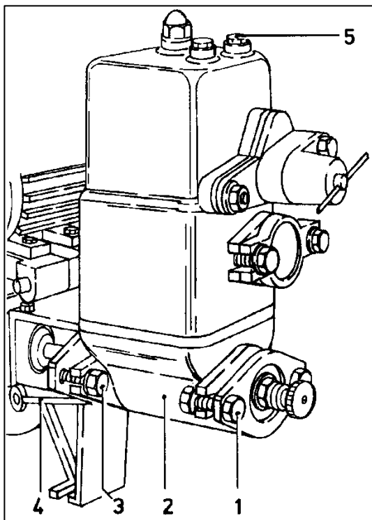
Abbildung 21: Pumpe entleeren
