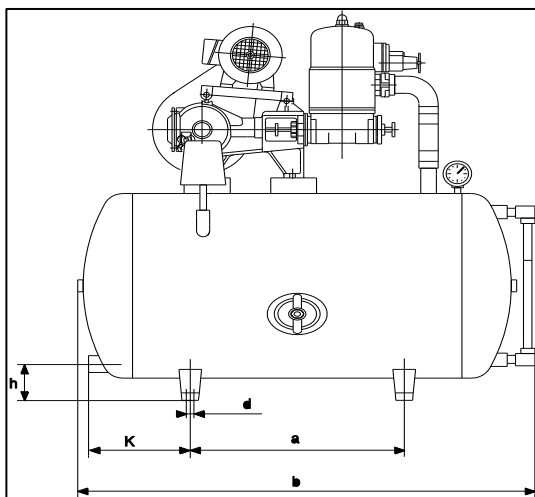
Abbildung 6: Maße in der Seitenansicht
