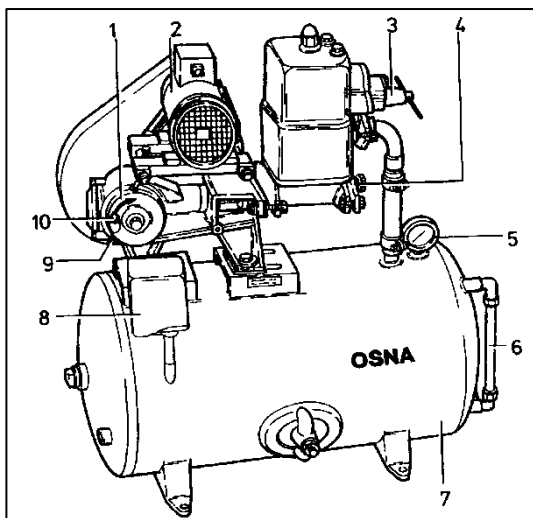
Abbildung 3: Funktionselemente 1
