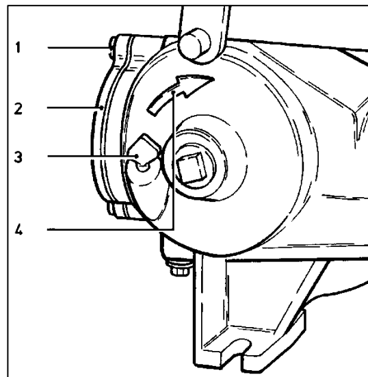
Abbildung 16: Antriebsgehäuse der Kolbenpumpe L
