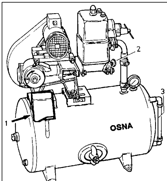
Abbildung 19: Druckschalter
