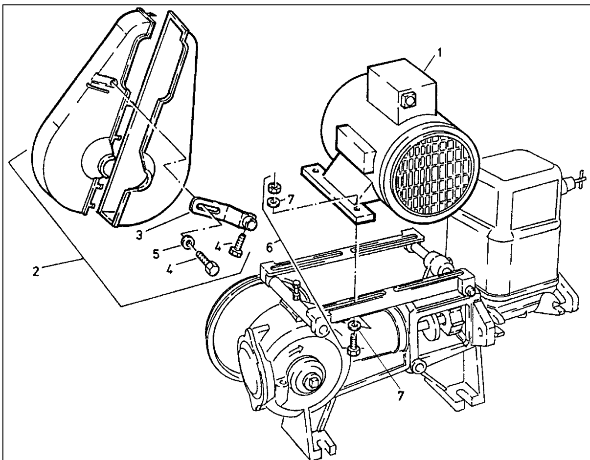
Abbildung 32: Explosionszeichnung Motoraufbau
