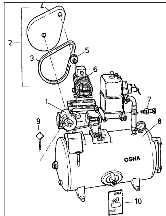
Abbildung 2: Lieferumfang Hauswasserautomat
