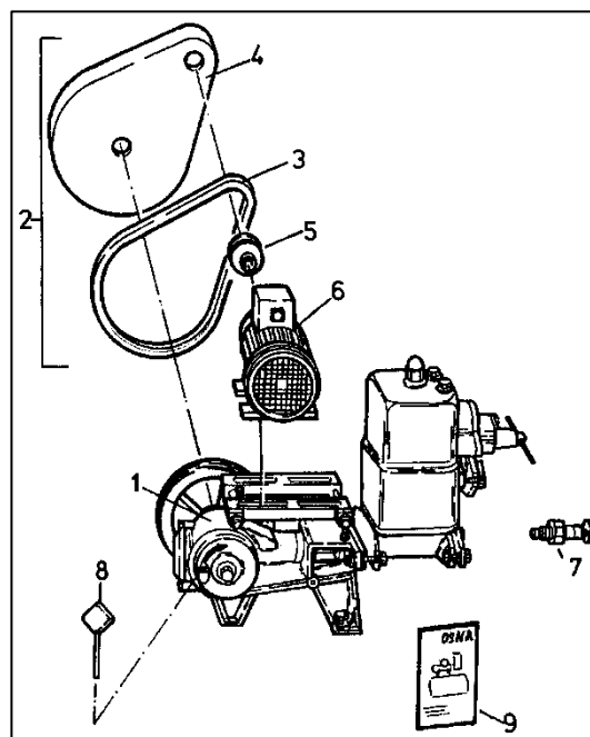
Abbildung 2: Lieferumfang Typ L
