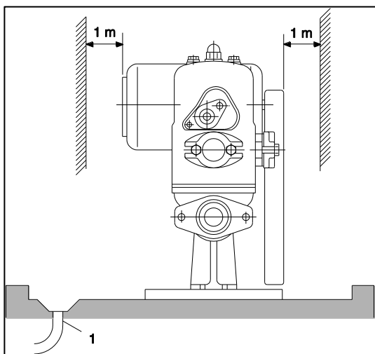
Abbildung 9: Aufstellraum Vorderansicht
