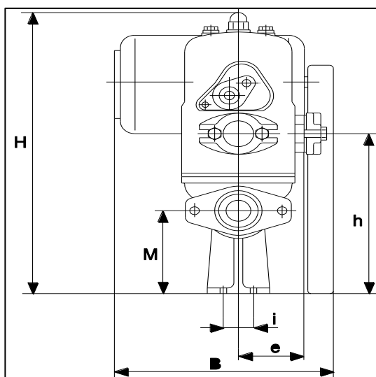
Abbildung 6: Maße in der Vorderansicht
