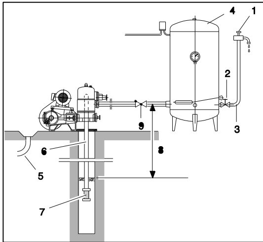
Abbildung 5: Aufbau mit Druckbehälter
