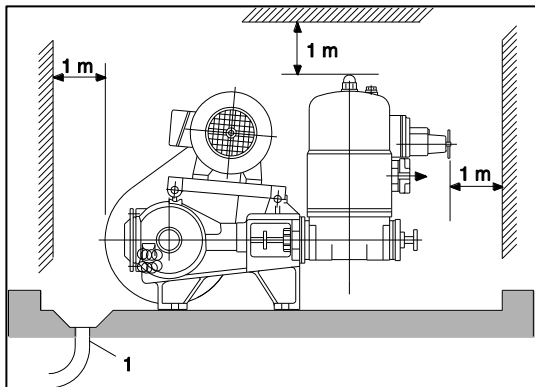
Abbildung 8: Aufstellraum Seitenansicht
