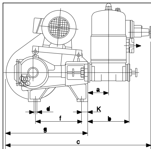
Abbildung 7: Maße in der Seitenansicht
