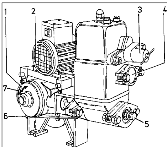
Abbildung 3: Funktionselemente 1
