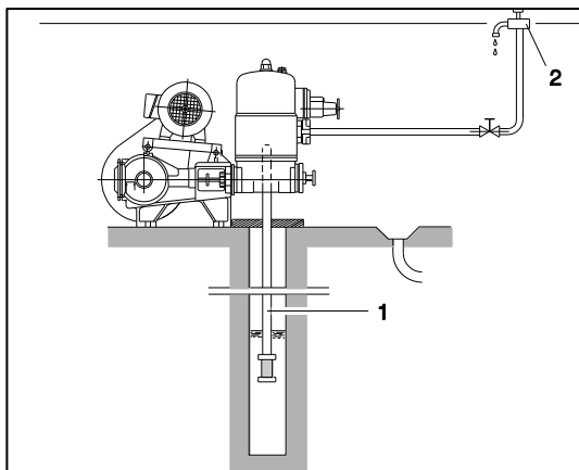
Abbildung 19: Anfahren der Kolbenpumpe
