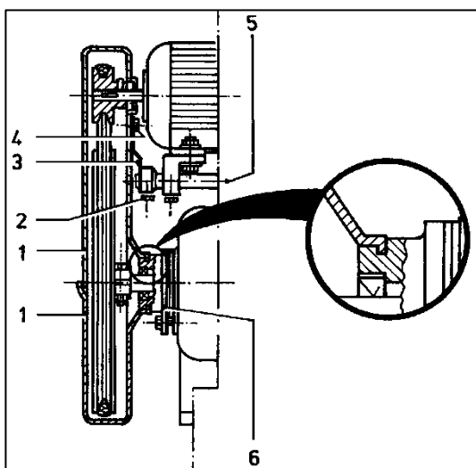
Abbildung 15: Riemenschutz
