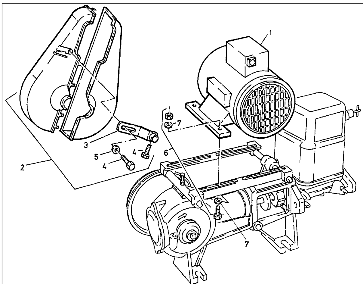
Abbildung 28: Explosionszeichnung Motoraufbau
