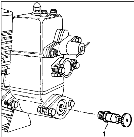
Abbildung 16: Schnüffelventil
