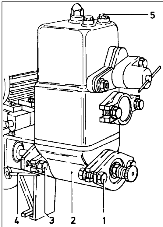
Abbildung 20: Pumpe entleeren
