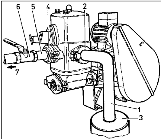
Abbildung 11: Wasseranschluss
