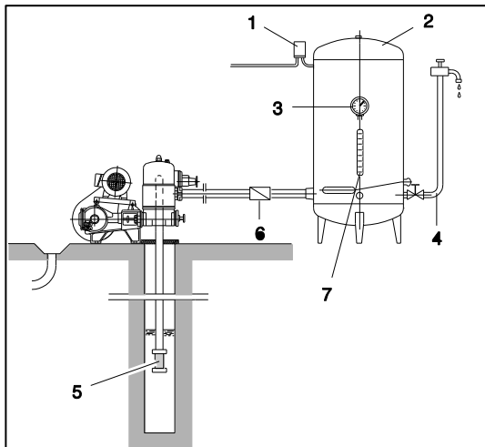
Abbildung 12: Aufstellung mit Druckbehälter
