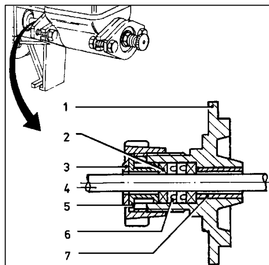
Abbildung 24: Stopfbuchse
