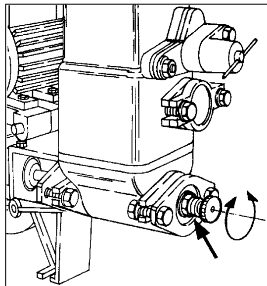
Abbildung 23: Luftpolsterergänzung
